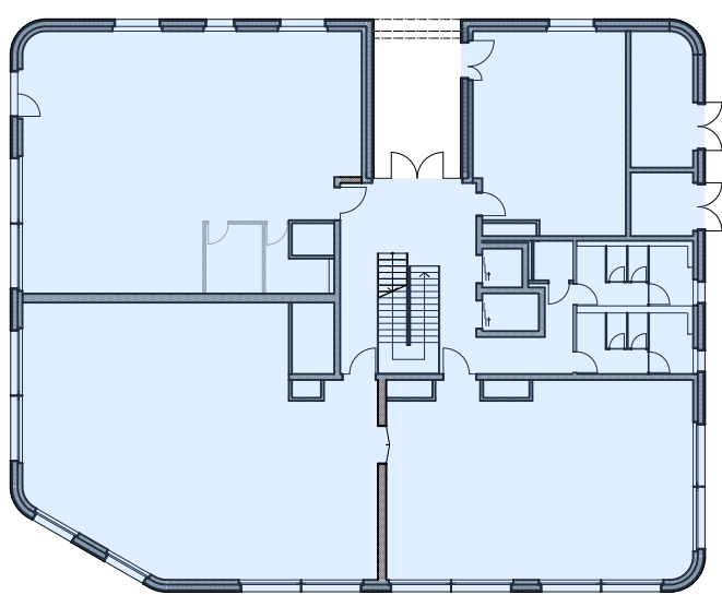
SCHEMA SURFACE DE PLANCHER
